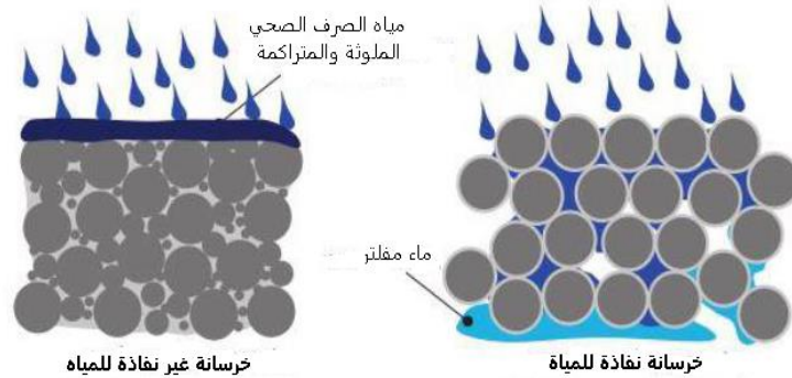
الشكل (1): الفرق بين الخرسانة النفاذة والخرسانة الغيرنفاذة
